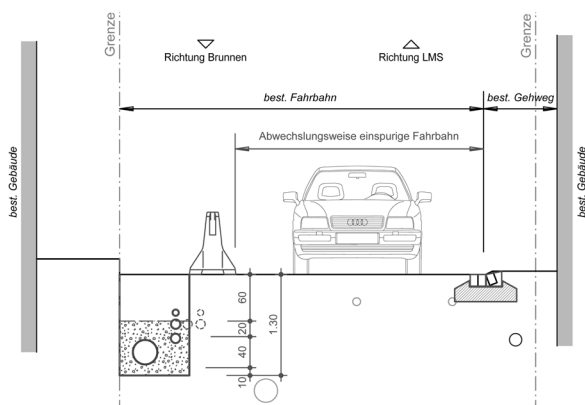
Normalprofil Regenabwasserleitung Dorfstrasse
