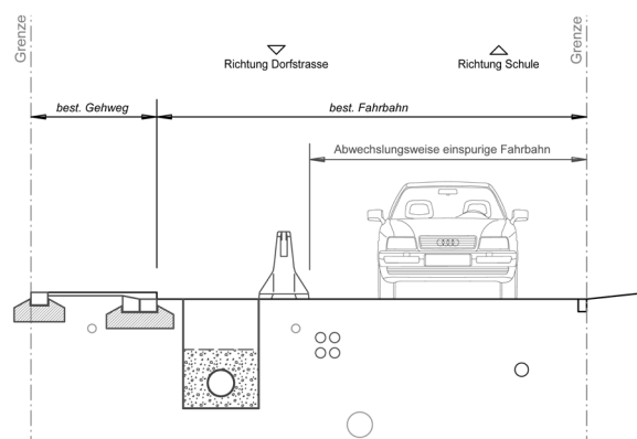
Normalprofil Regenabwasserleitung Schulstrasse
