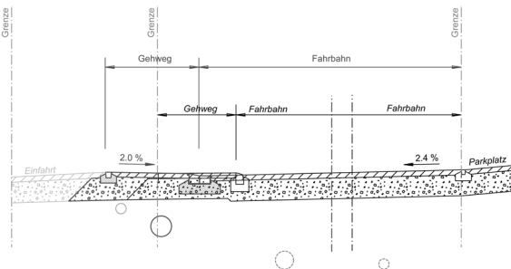
Normalprofil Regenabwasserleitung Axensteinstrasse
